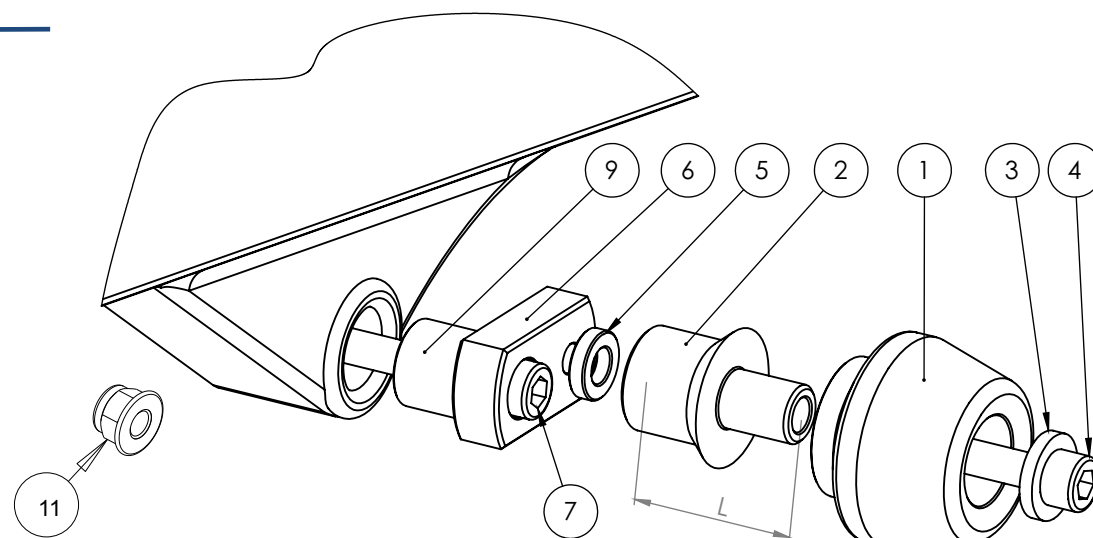
Wymiary tulejek
